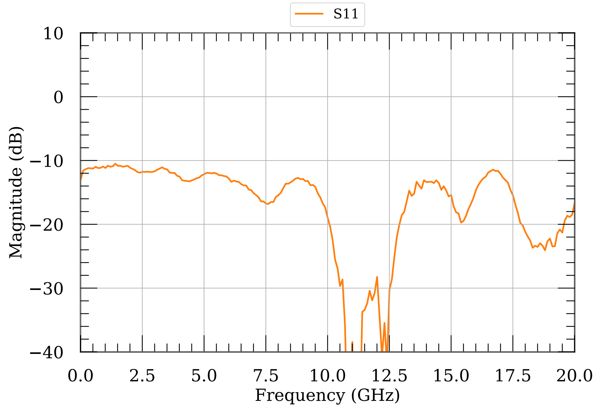
LNA S-params module076v2
